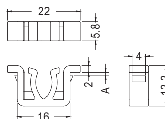
門扣本體
