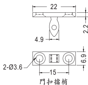
門扣擋梢
